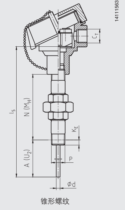
“螺纹短节-活接头-螺纹短节” 式颈管
