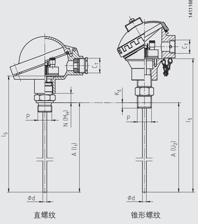
双螺纹六角头套管 (带六角头扳手卡口)
