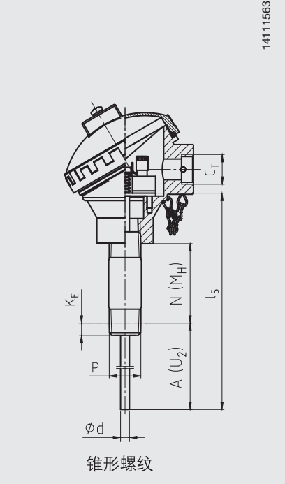
双螺纹六角头套管 (管道部分)
